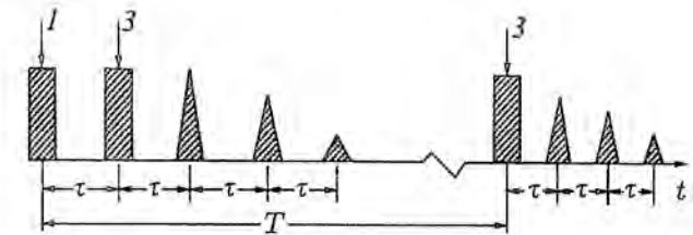
Fig. 3.11. Cyclotron echo.
