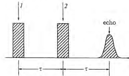
Fig. 3.8. Spin echo.
